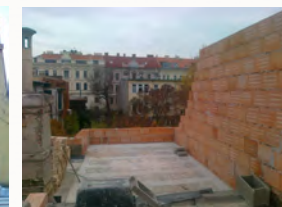
Aufmauern des Kniestocks für den Betonrost
